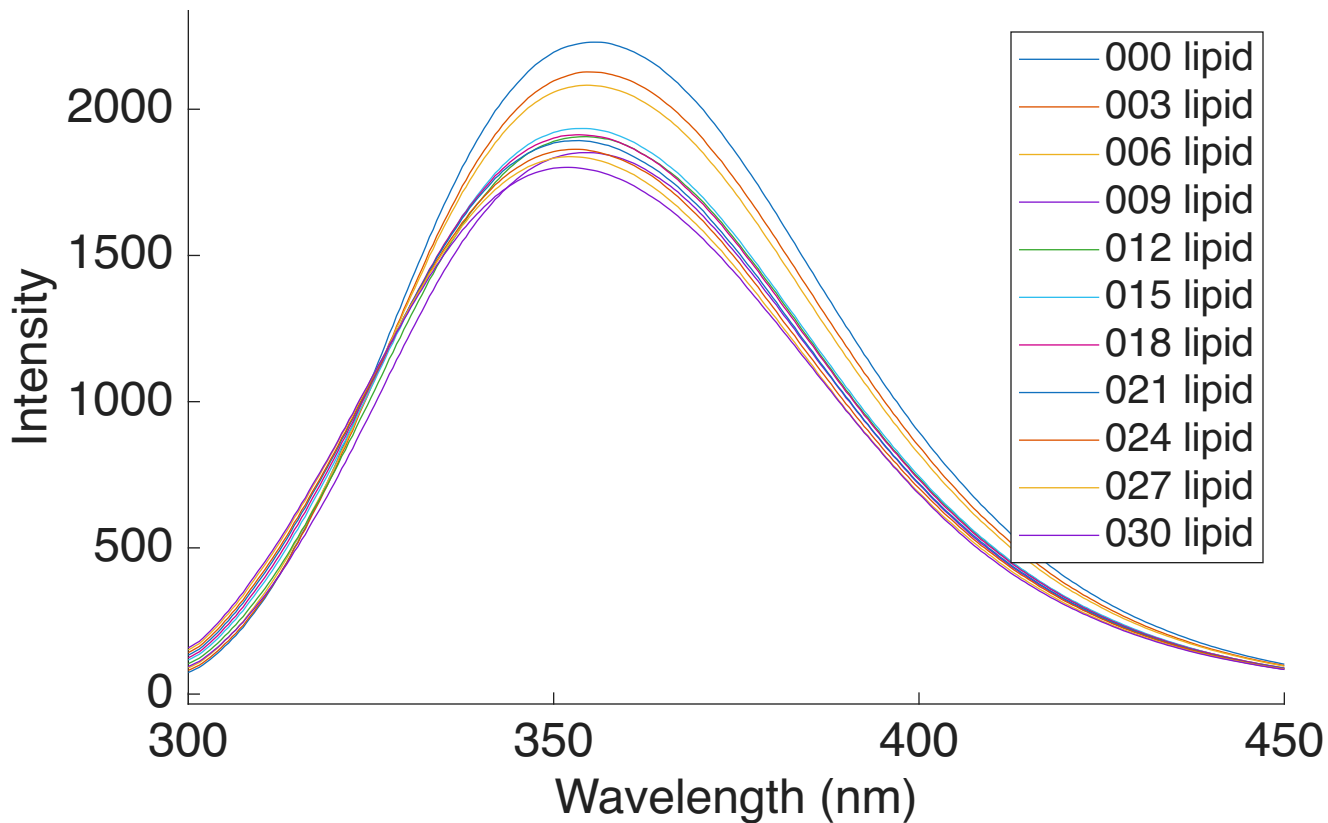
BFI titration - no corrections
